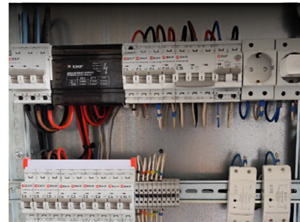
ВА 47-63N 6кА Автоматический выключатель РДЕ-47 16А Розетка АВДТ-63N Автоматический выключатель дифференциального тока
