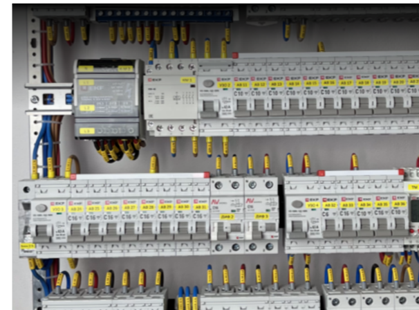
ВН-63N Выключатель нагрузки ВА 47-63N 6кА Автоматический выключатель ВД-100N Выключатели дифференциального тока (УЗИП) ОПВ Класс 2 Автоматический выключатель дифференциального тока КМ Контактный модульный
