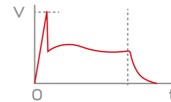
Форма импульса напряжения при срабатывании УЗИП комбинированного типа
