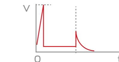
Форма импульса напряжения при срабатывании УЗИП коммутирующего типа
