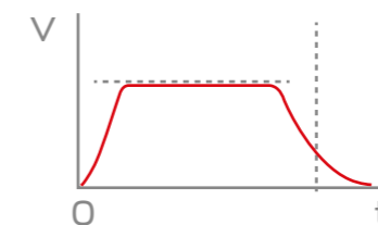
Форма импульса напряжения при срабатывании УЗИП ограничивающего типа
