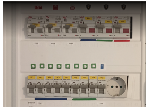
ВН-63N Выключатель нагрузки ВА 47-63N 6кА Автоматический выключатель РДЕ-47 16А Розетка
