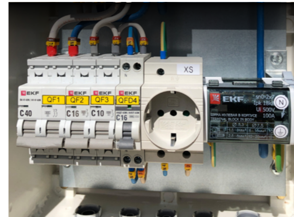
ВА 47-63N 6кА Автоматический выключатель АВДТ-63М Автоматический выключатель дифференциального тока РДЕ-47 16А Розетка
