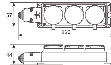
Колодка 3-х гнездная удлинителя-шнура
